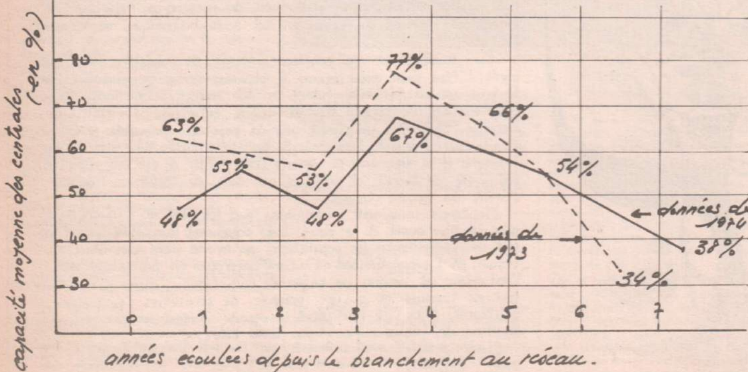
Facteur de capacité des centrales en fonction de leur âge
